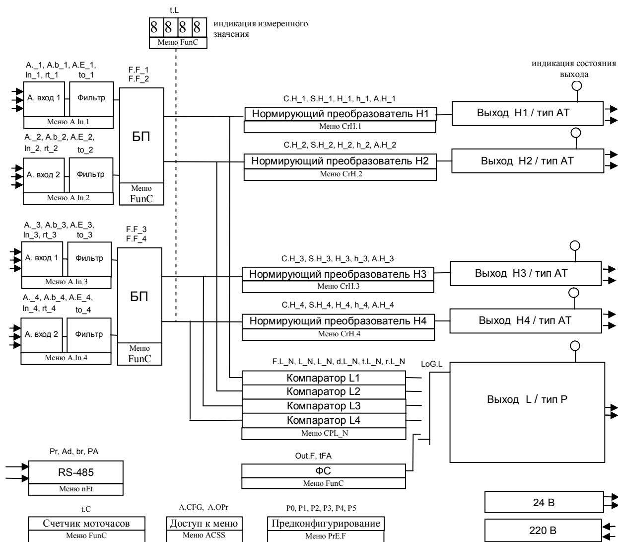
Рисунок 4 – Функциональная структура приборов М-1745-4АТ
