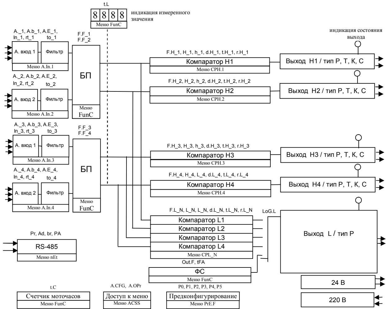
Рисунок 2 – Функциональная структура приборов М-1745- 4Р, 4Т, 4К, 4С
