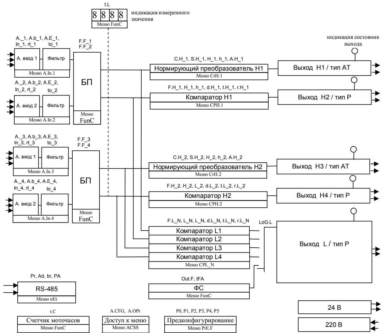
Рисунок 3 – Функциональная структура приборов М-1745-2АТ/2Р
