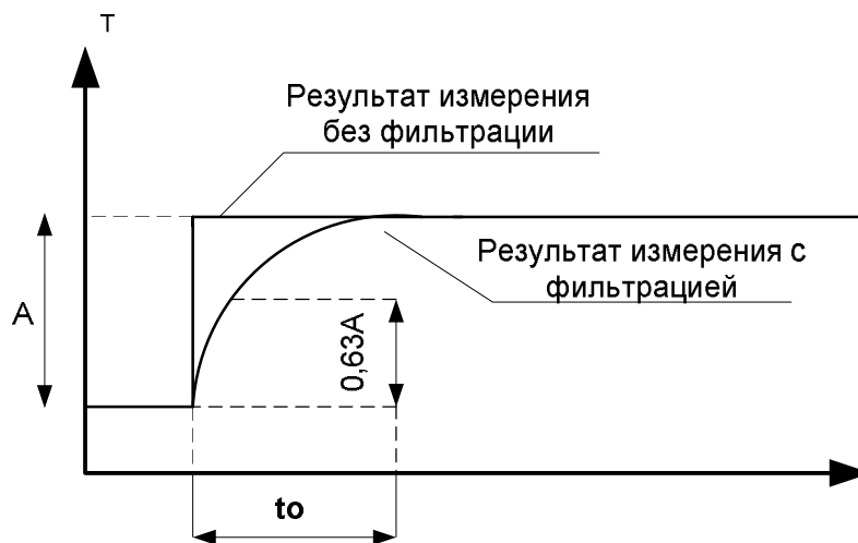
Рисунок 5 – Цифровая фильтрация результата измерения
