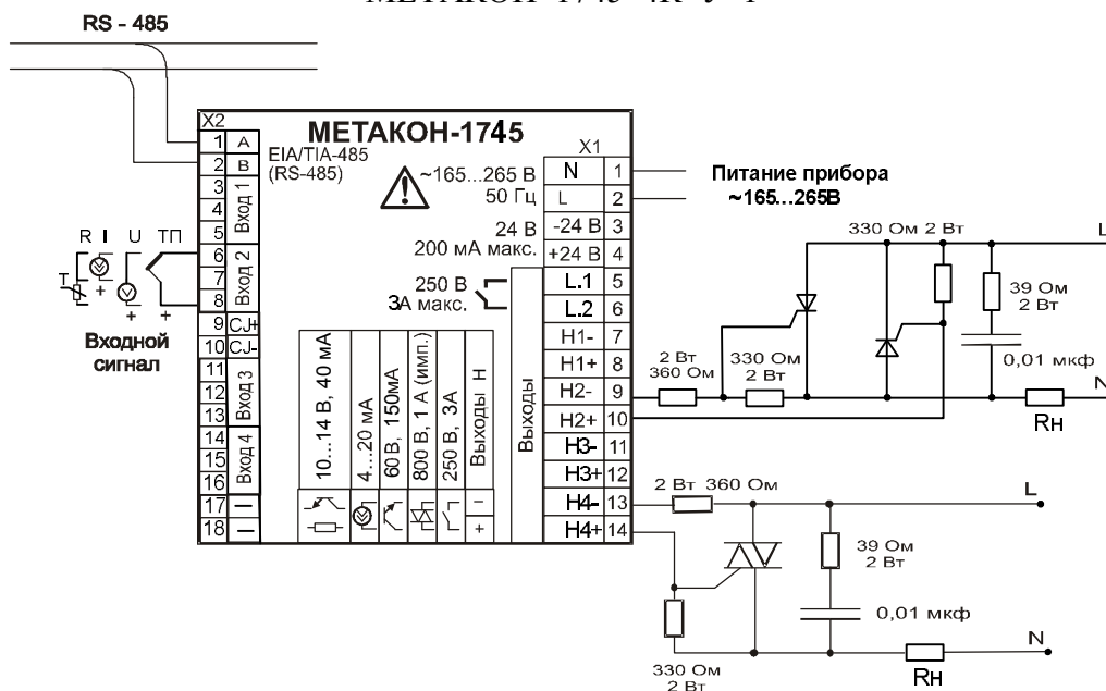
Рисунок 13 – Электрическая схема подключения внешнего симистора и тиристоров к прибору МЕТАКОН-1745-4С-У-1
