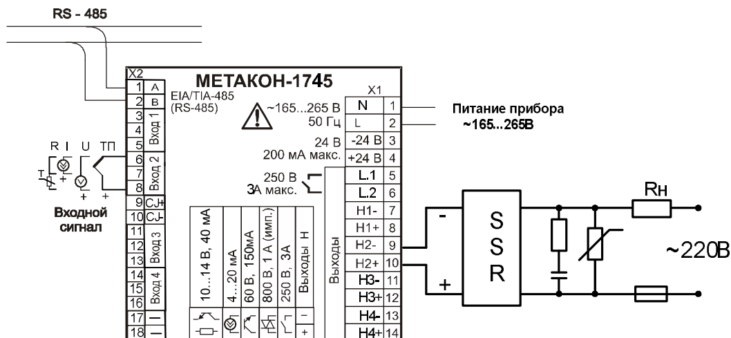
Рисунок 12 – Электрическая схема подключения твердотельного реле к прибору МЕТАКОН-1745-4К-У-1
