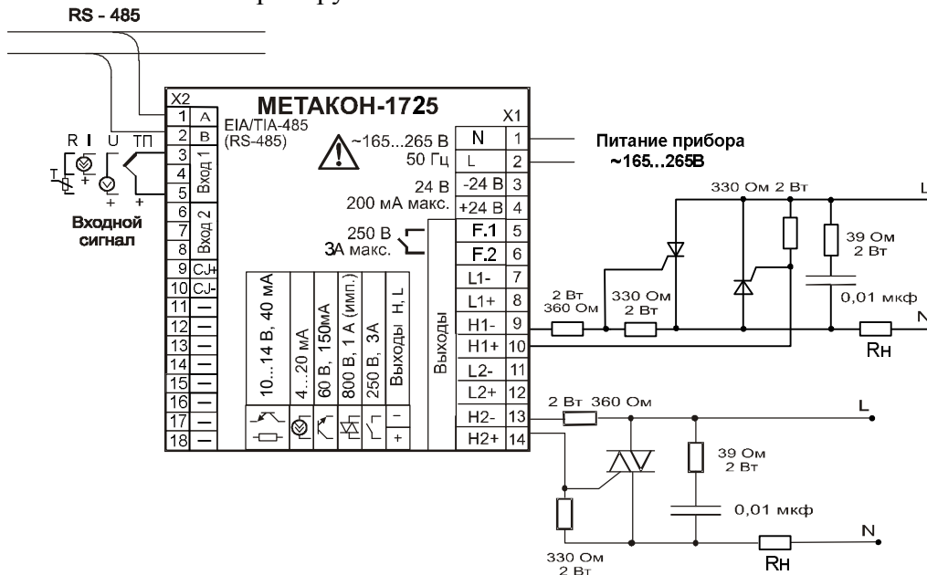
Рисунок 13 – Электрическая схема подключения внешнего симистора и тиристора к прибору МЕТАКОН-1725-2С/2Р-У-1
