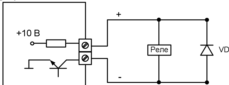
Рисунок 17 – Схема подключения электромагнитного реле к выходу типа «К»
