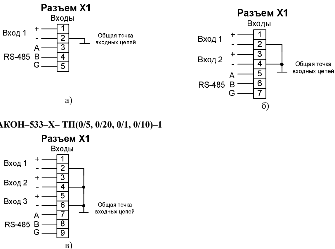
Рисунок 8 – Схемы подключения входных сигналов к клеммным соединителям для мод. МЕТАКОН-5Х3-Х-ТП(0/5, 0/20, 0/1, 0/10)–1
