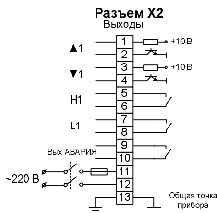
Рисунок 15 – Схемы подключения выходных цепей к клеммным соединителям для модификаций МЕТАКОН-513-КР-Х-Х
