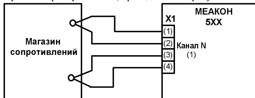
Рисунок А.6.4.2.1– Схема подключения приборов мод. МЕТАКОН 5ХХ для проведения поверки по входным сигналам сопротивления
