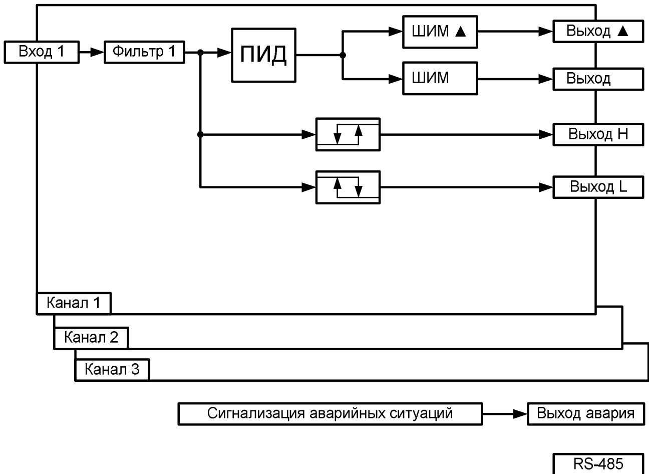
Рисунок 1 – Функциональная схема прибора МЕТАКОН-5х3-Х-Х-Х
